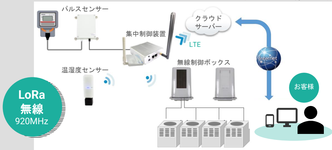
無線とソーラー発電を使用したデマンドシステム(特許7085069号)
